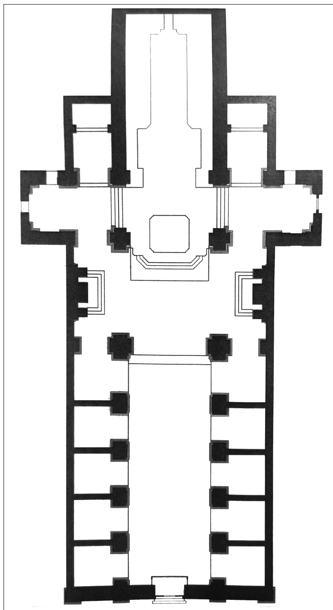
Fig. 1. San Martino delle Scale (Palermo), chiesa abbaziale; pianta (elaborazione grafica di Simona Silvia).
